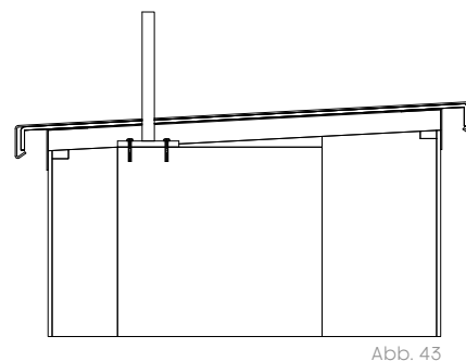
fenorm Aluminium Mauerabdeckung mit Durchdringung für Geländer
