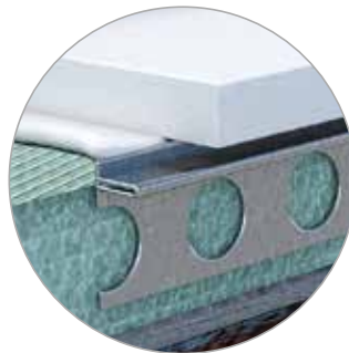
Einbau bei Ziegelparapet mit verputzter Fläche
