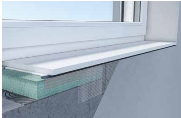
Einbau bei Betonparapet mit verspachtelter Oberfläche
