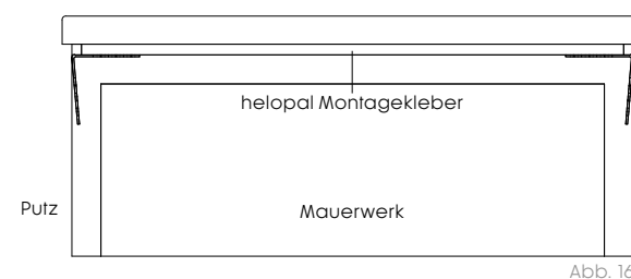
Mauerabdeckung linea mit wenig Überstand
