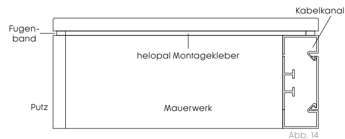
Mauerabdeckung linea mit Kabelkanal / Fugenband
