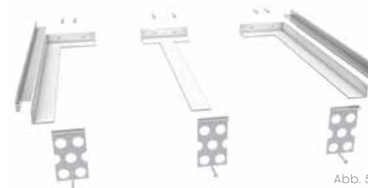
Einbau mit Montageset - passend für Schattennutprofil 4 und 5 mm (Erweiterungsset für Fensterbänke ab 1,50 m erhältlich)
