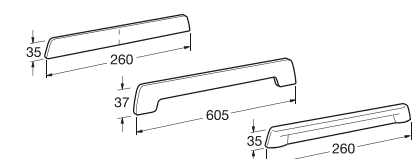
exclusiv Abschlusskappen
