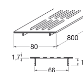
Lüftungsgitter
