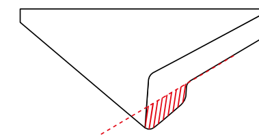
Vorderkante bündig fräsen****
