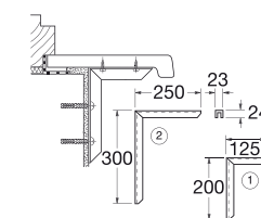
Konsolen
