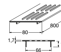
Lüftungsgitter
