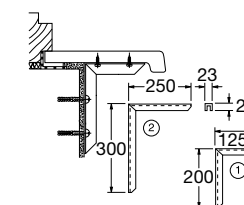
Konsolen
