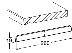
Abschlusskappen
