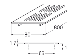
Lüftungsgitter
