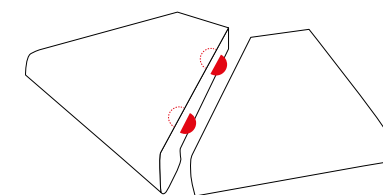
Gehrungsverbindung mit Lamellos**
