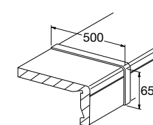
Fensterbank- Verbindungsprofile
