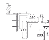
Konsolen
