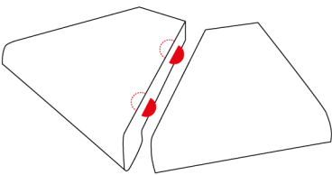
Gehrungsverbindung mit Lamellos**
