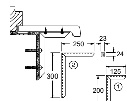
Konsolen
