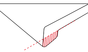
Vorderkante bündig fräsen****
