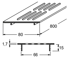
Lüftungsgitter
